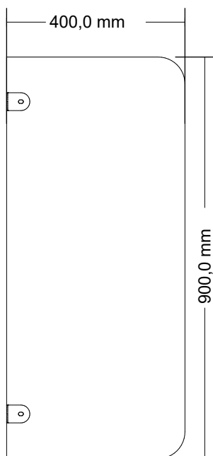
PROSPETTO LATERALE
